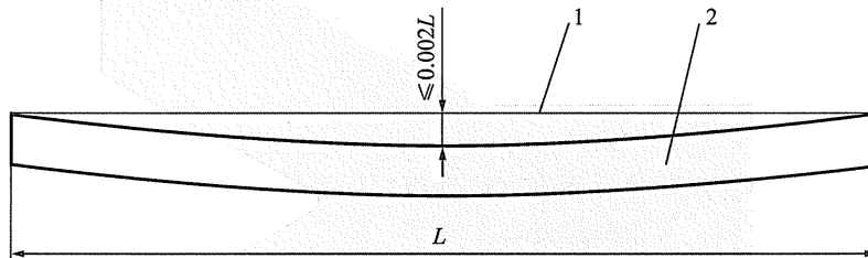
1—拉紧的线或钢丝；2—钢管
