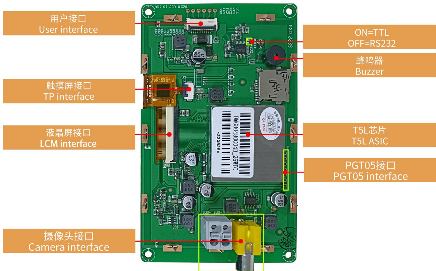
硬件接口图
